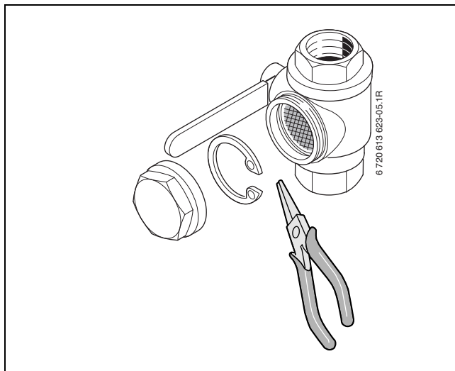
Kuva 31 Lukkorengaalla varustettu suodatinvaihtoehto
