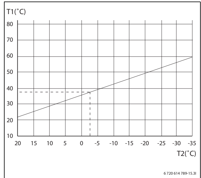
Kuva 21 Lämpöpatteri
