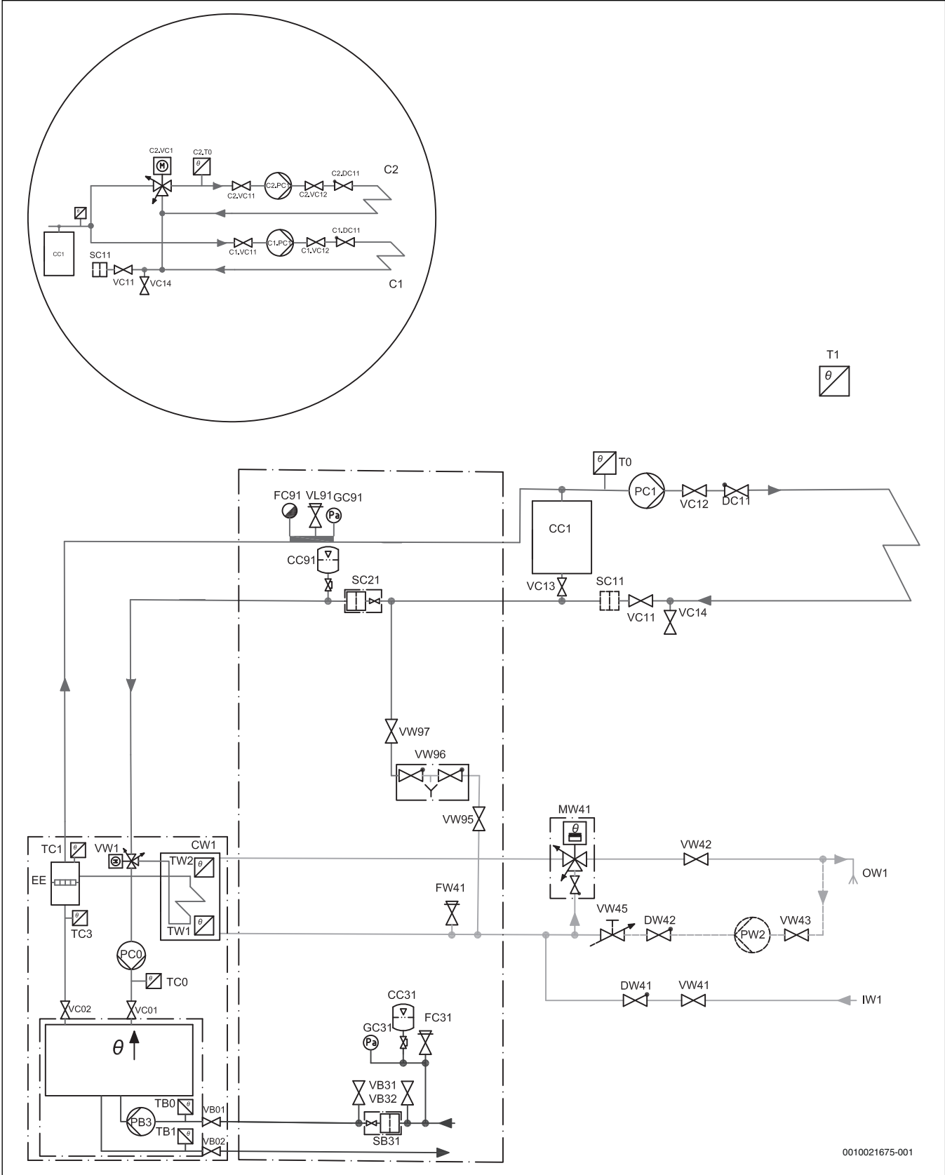
Kuva 46 Puskurivaraaja
