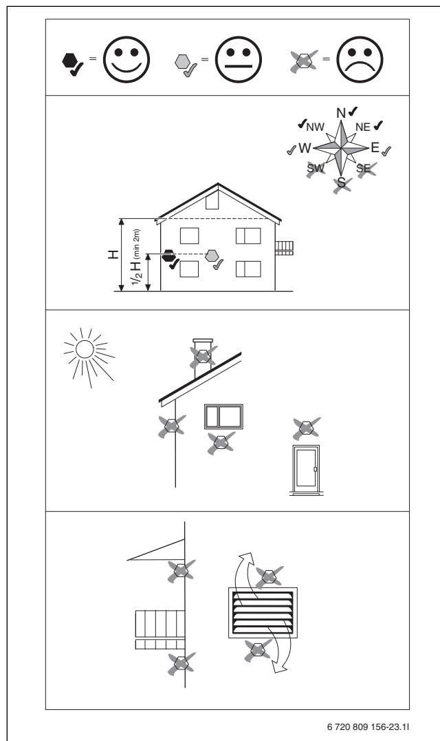
Kuva 18 Ulkolämpötila-anturin sijoituspaikka
