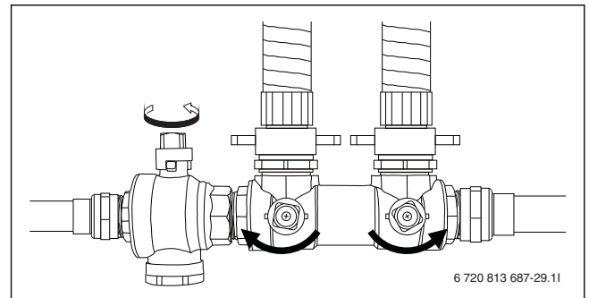
Kuva 25 Täyttöyksiköt täyttöasennossa
