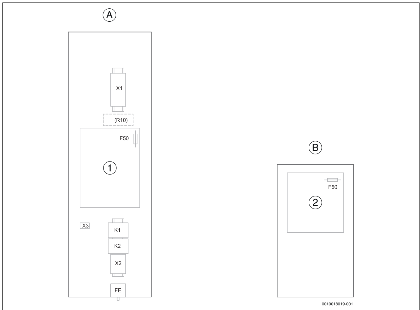
Kuva 48 Sähkörasioiden yhteenveto
