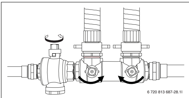
Kuva 29 Täyttöyksiköt normaaliasennossa
