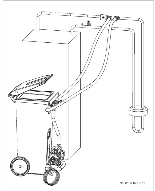
Kuva 24 Täyttöasemasta täyttäminen
