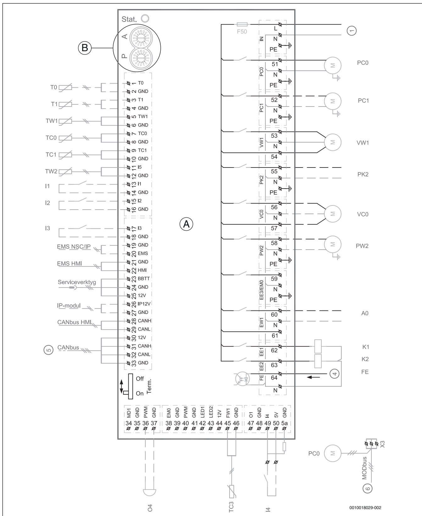
Kuva 51 Sähköpiirikaavio asentajamoduuli
