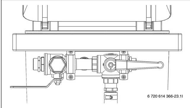
Kuva 27 Täyttöasema täyttöasennossa
