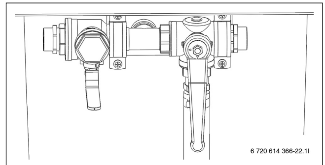
Kuva 26 Täyttöasema sekoitusasennossa
