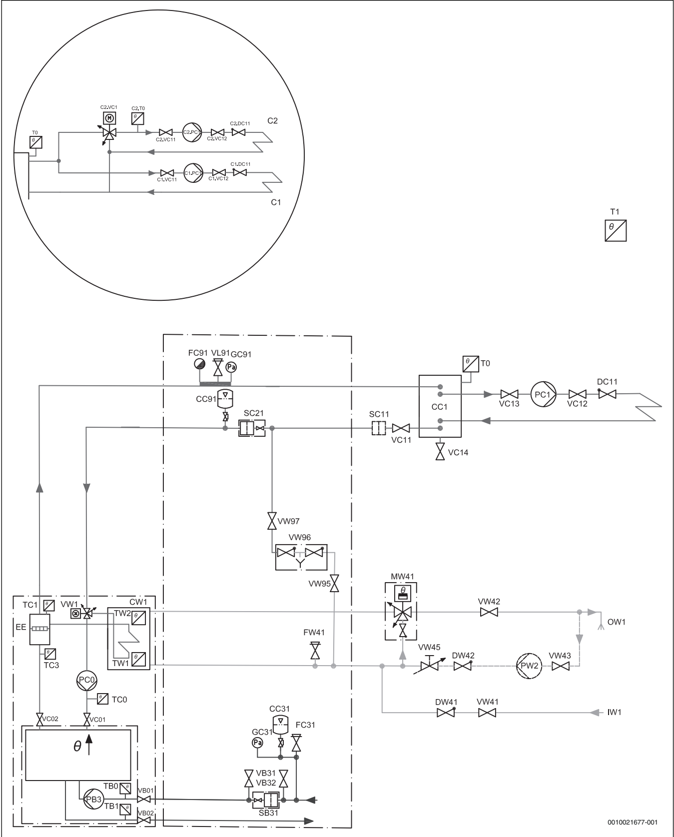
Kuva 47 Puskurivaraaja samansuuntainen
