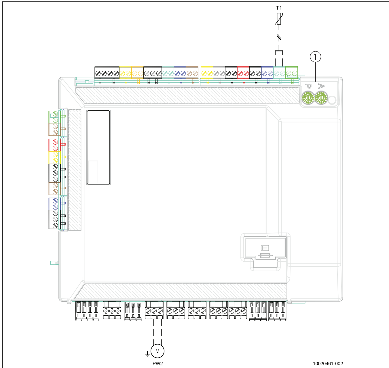
Kuva 15 Liitännät asennusmoduulissa
