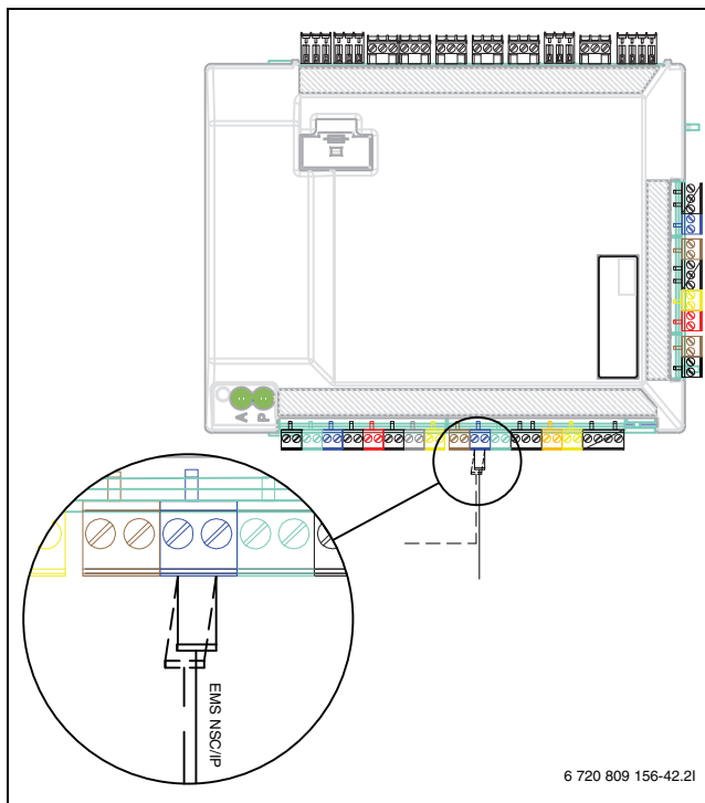
Kuva 45 EMS-liitäntä asennusmoduulissa
