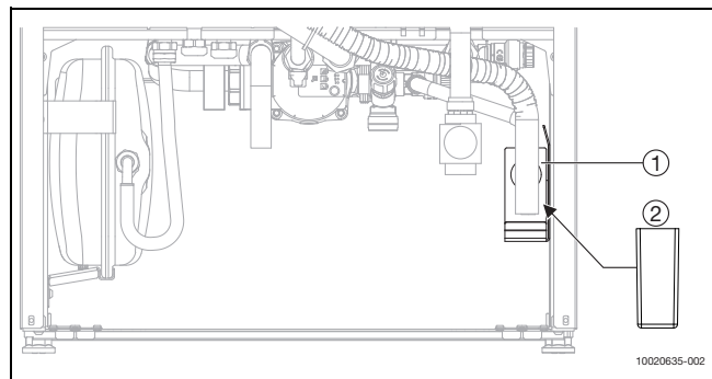
Kuva 5 Vuotovesisäiliön liitäntäalue
