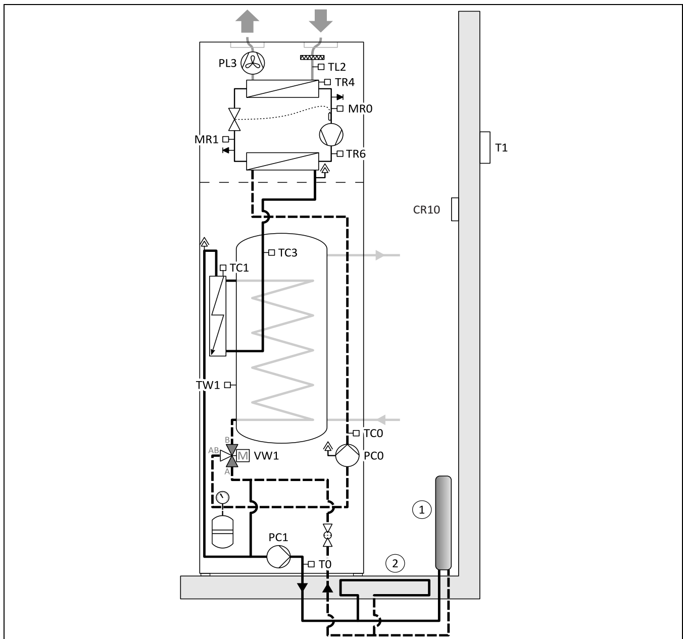
Kuva 29 Toiminnallinen yleiskuvaus
