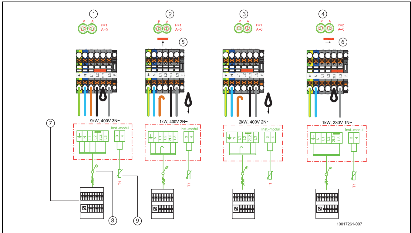
Kuva 14 Ulkoiset liitännät 1-9 kW
