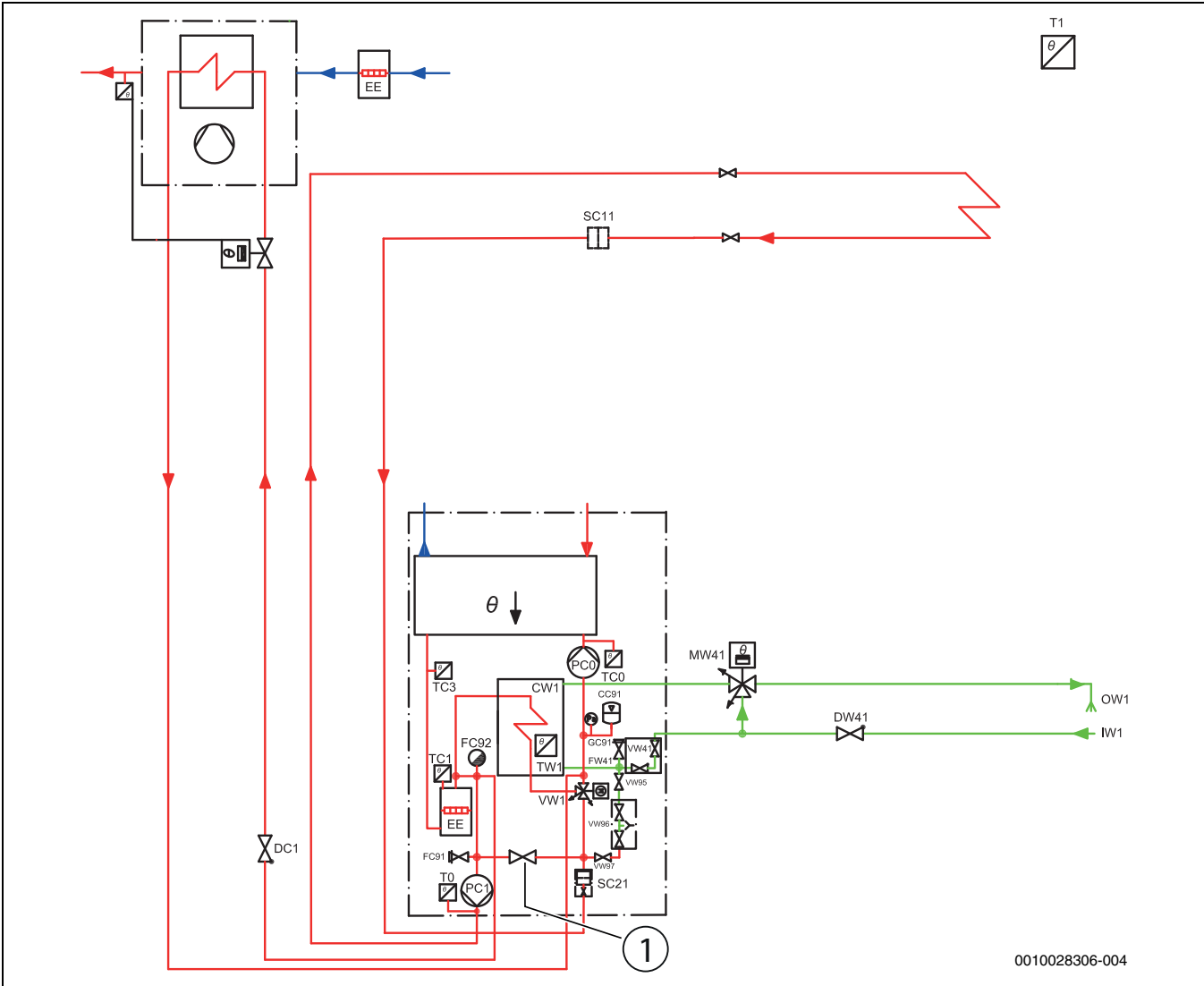
Kuva 36 Tuloilman lämmitys, lämmityspiiri sekoitusventtiilin kanssa ja ilman sitä
