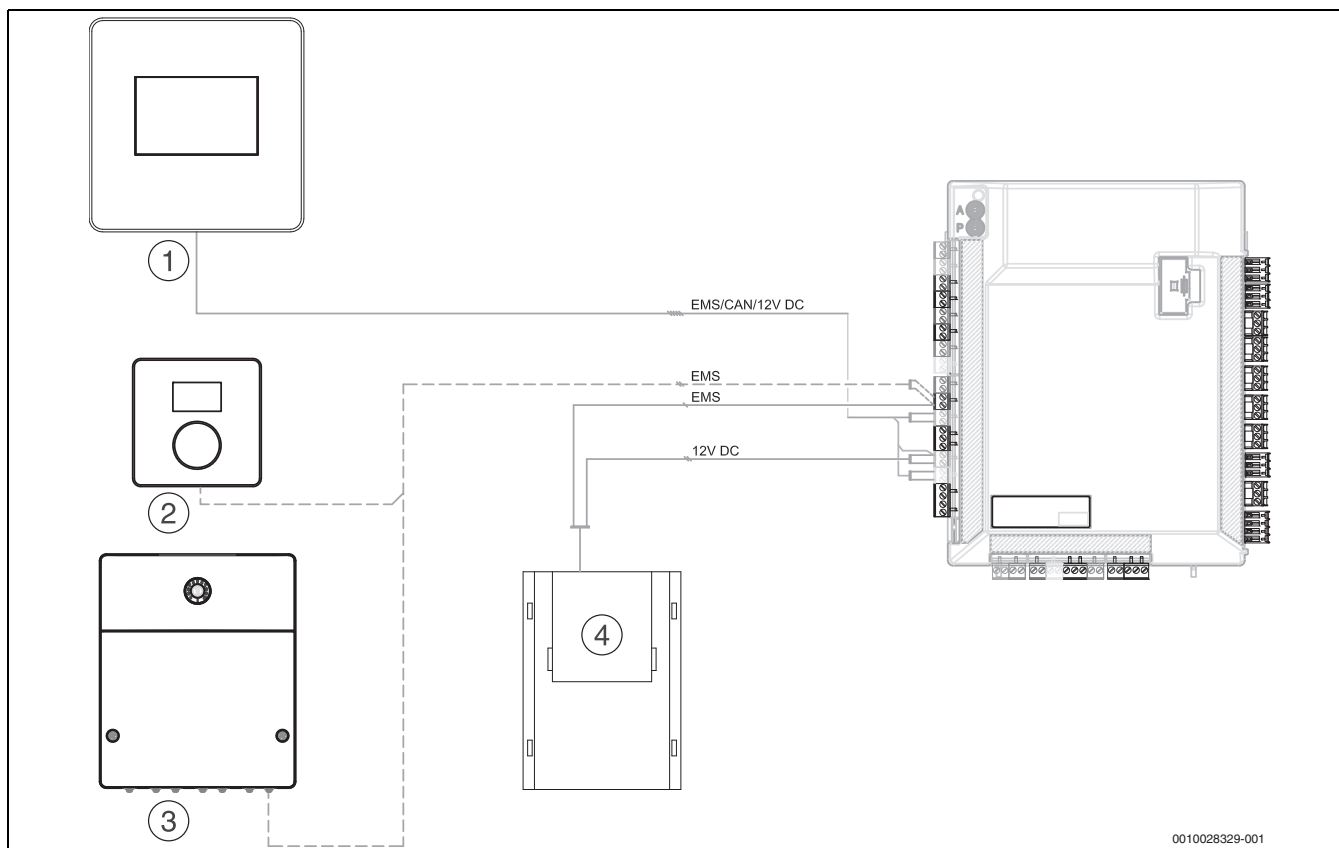
Kuva 41 Sähköpiirikaavio EMS väylä
