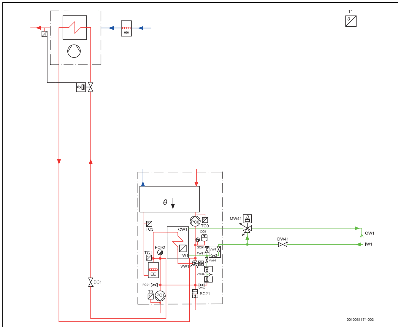
Kuva 35 Tuloilmalämmittin ilman lämmityspiiriä
