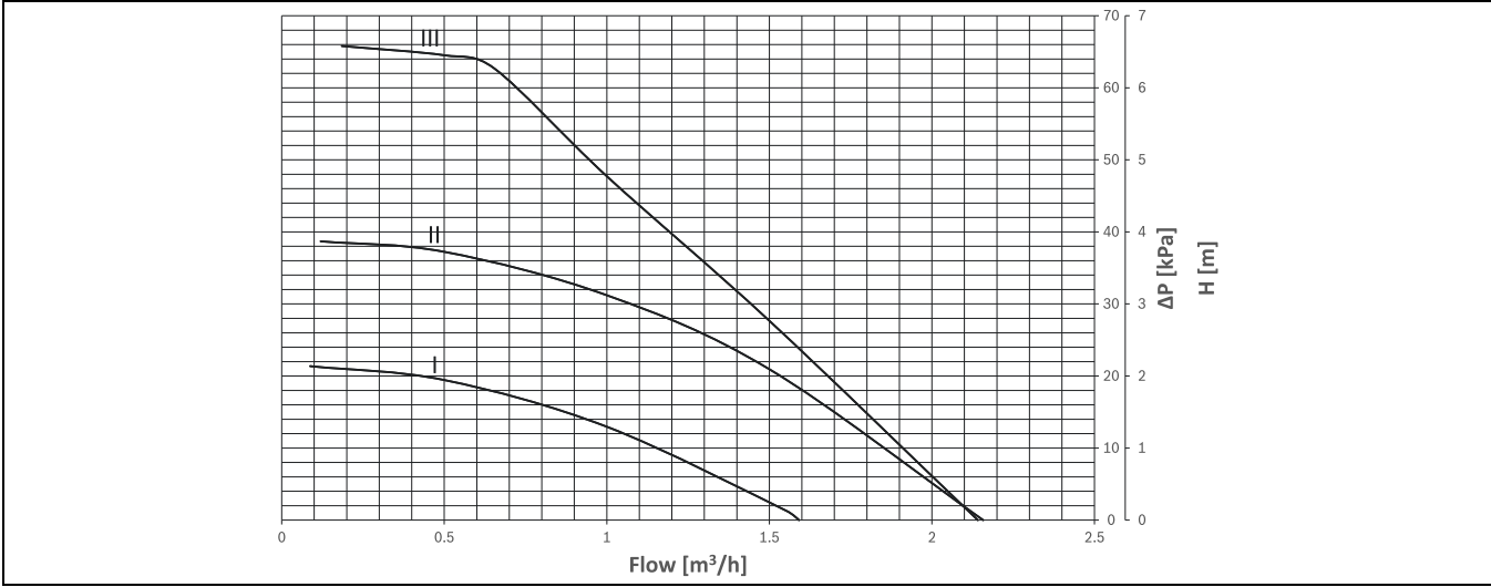
Kuva 32 Virtauskaavio – Lämmönsiirtonestepumppu
