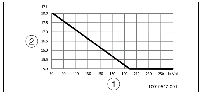
Kuva 17 Alhaisin imuilman lämpötila kompressorin käytölle
