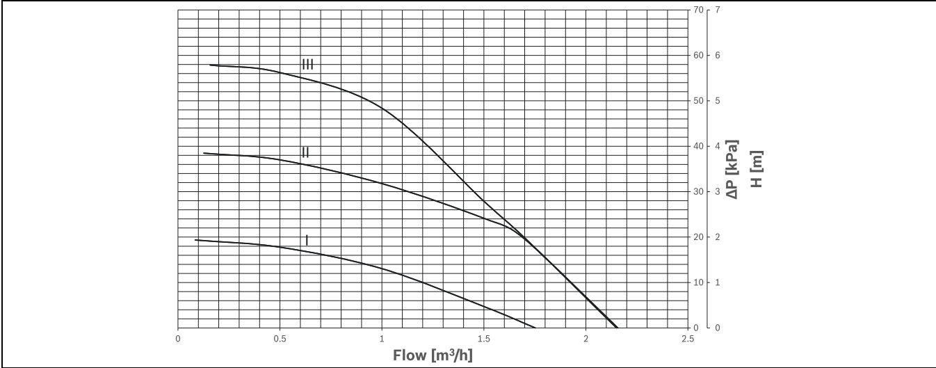
Kuva 31 Virtauskaavio – Lämmönsiirtonestepumppu
