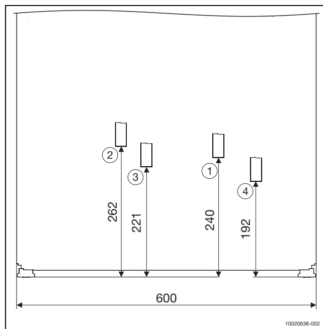
Kuva 11 Putkiliitännöjen kuva edestä
