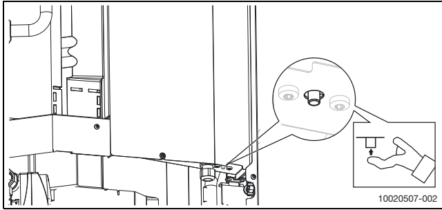
Kuva 20 Liitäntäkotelon alapuolella olevan termostaattipainikkeen sijainti.
