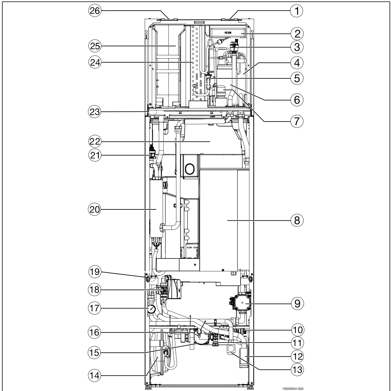
Kuva 2 Rakennneosat
