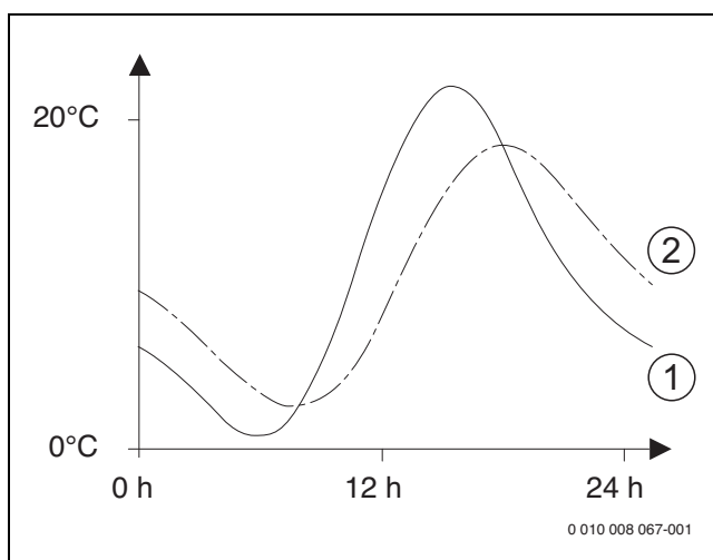
Kuva 18 Esimerkki ulkoilman lämpötilan kompensoinnista:
