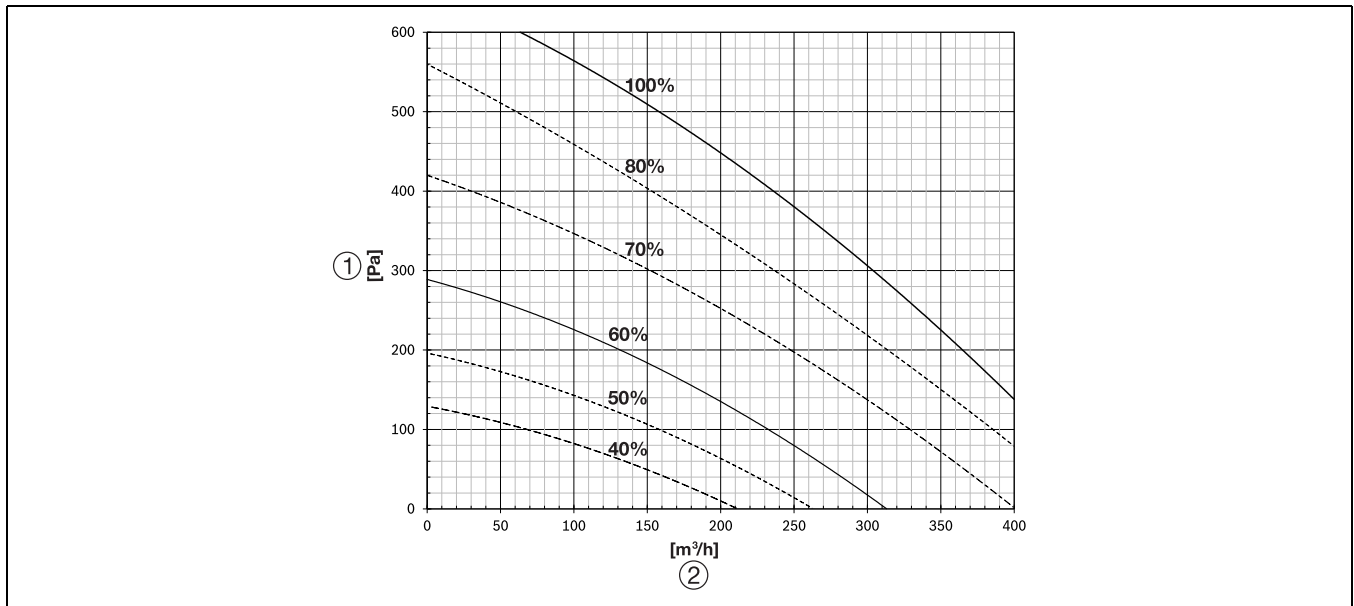
Kuva 33 Kaavio - paine / ilmavirta
