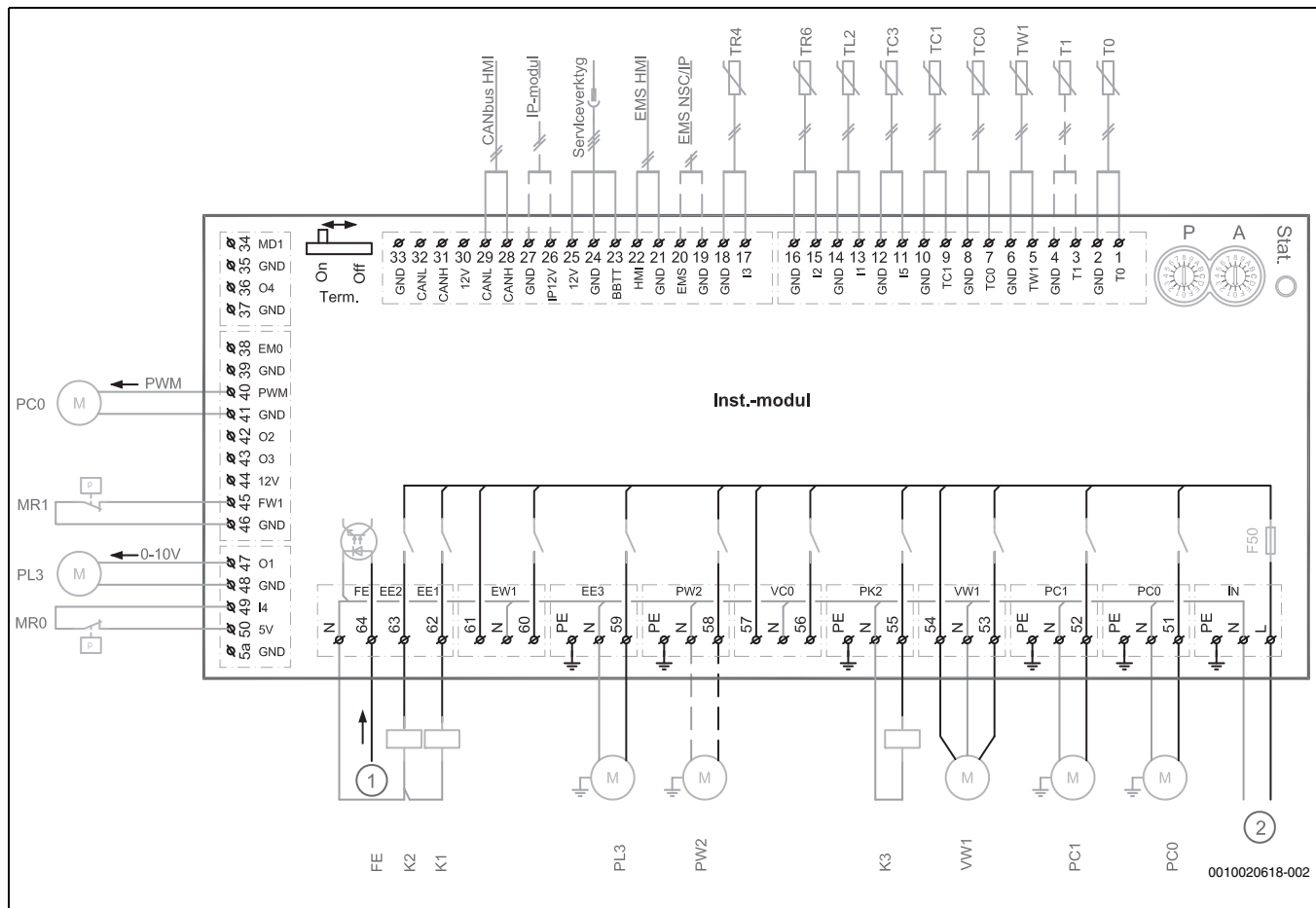
Kuva 40 Asentajamoduulin sähköpiirikaavio
