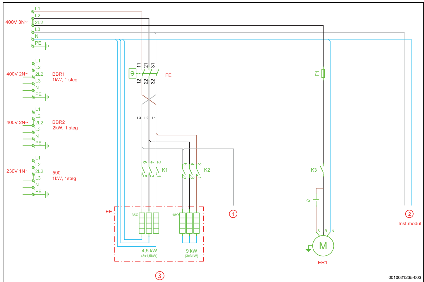
Kuva 39 Päävirtapiirin kytkentäkaavio, 400 V 3N
