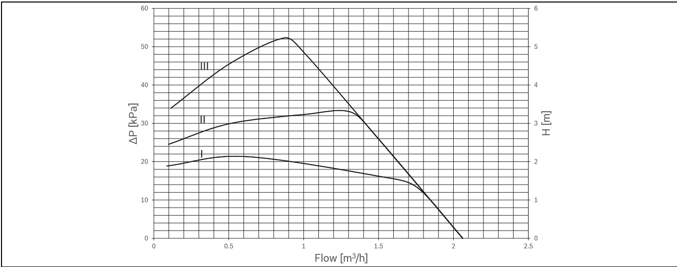
Kuva 30 Virtauskaavio – Lämmönsiirtonestepumppu
