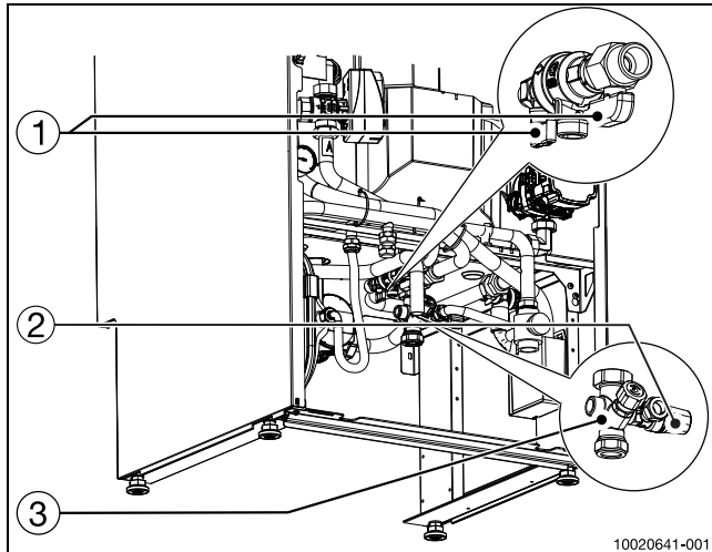
Kuva 28 Lämminvesivaraajan tyhjennys
