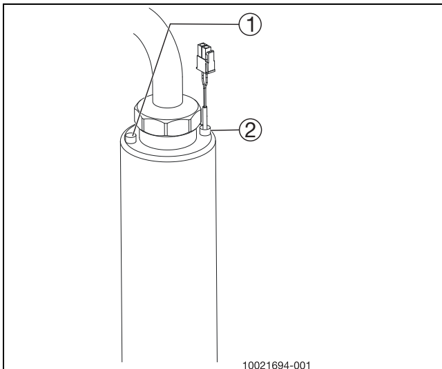
Kuva 21 Upotettava pidike anturille
