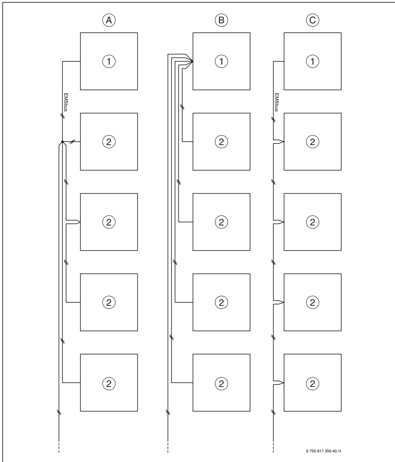
Kuva 42 Liitännävaihtoehto EMS-väylä
