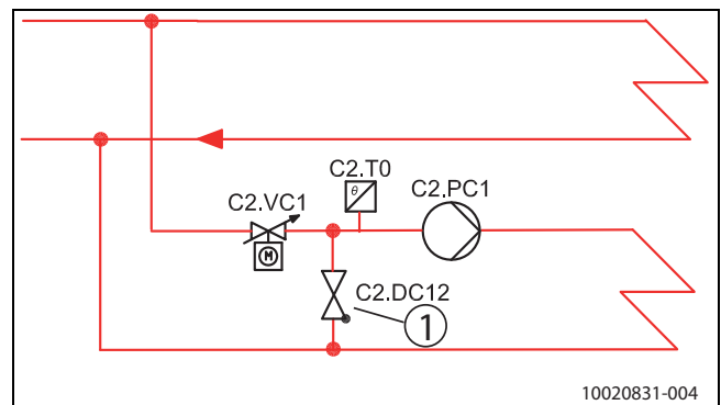
Kuva 34 Lämmityspiiri 2
