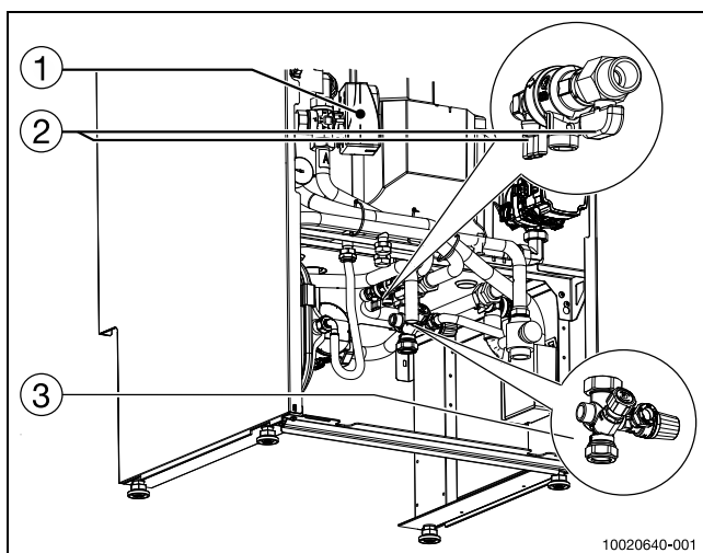
Kuva 16 Hydraulikkaliitännät
