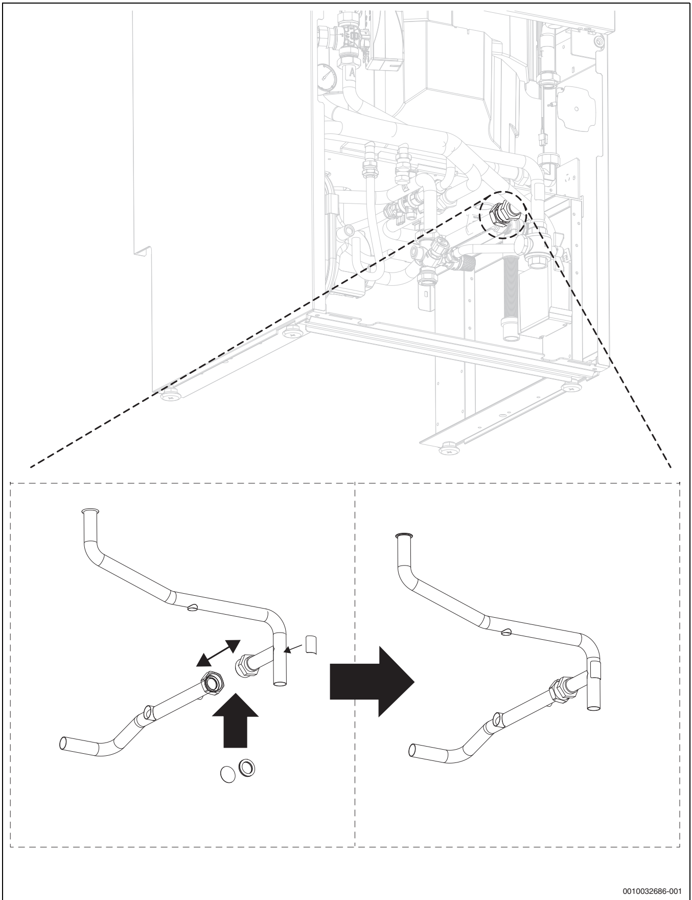
Kuva 38 Ohituspysäytä sulkulevyillä
