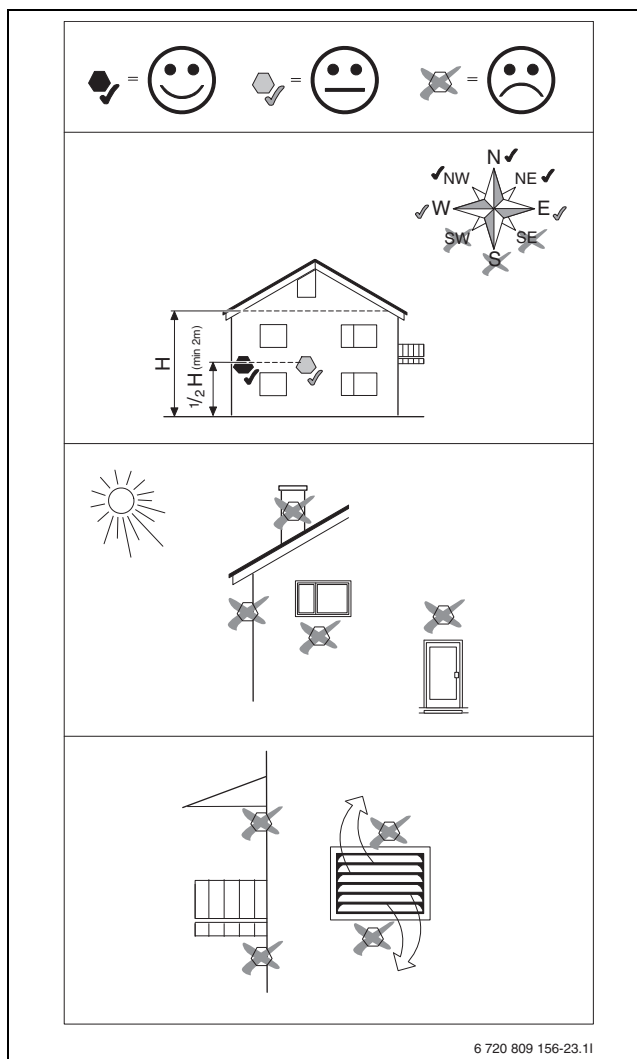
Kuva 13 Ulkolämpötila-anturin asennus
