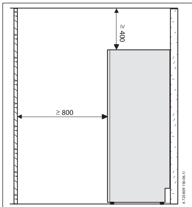
Kuva 5 Lämpöpumpputuotteen vähimmäisetäisyys
