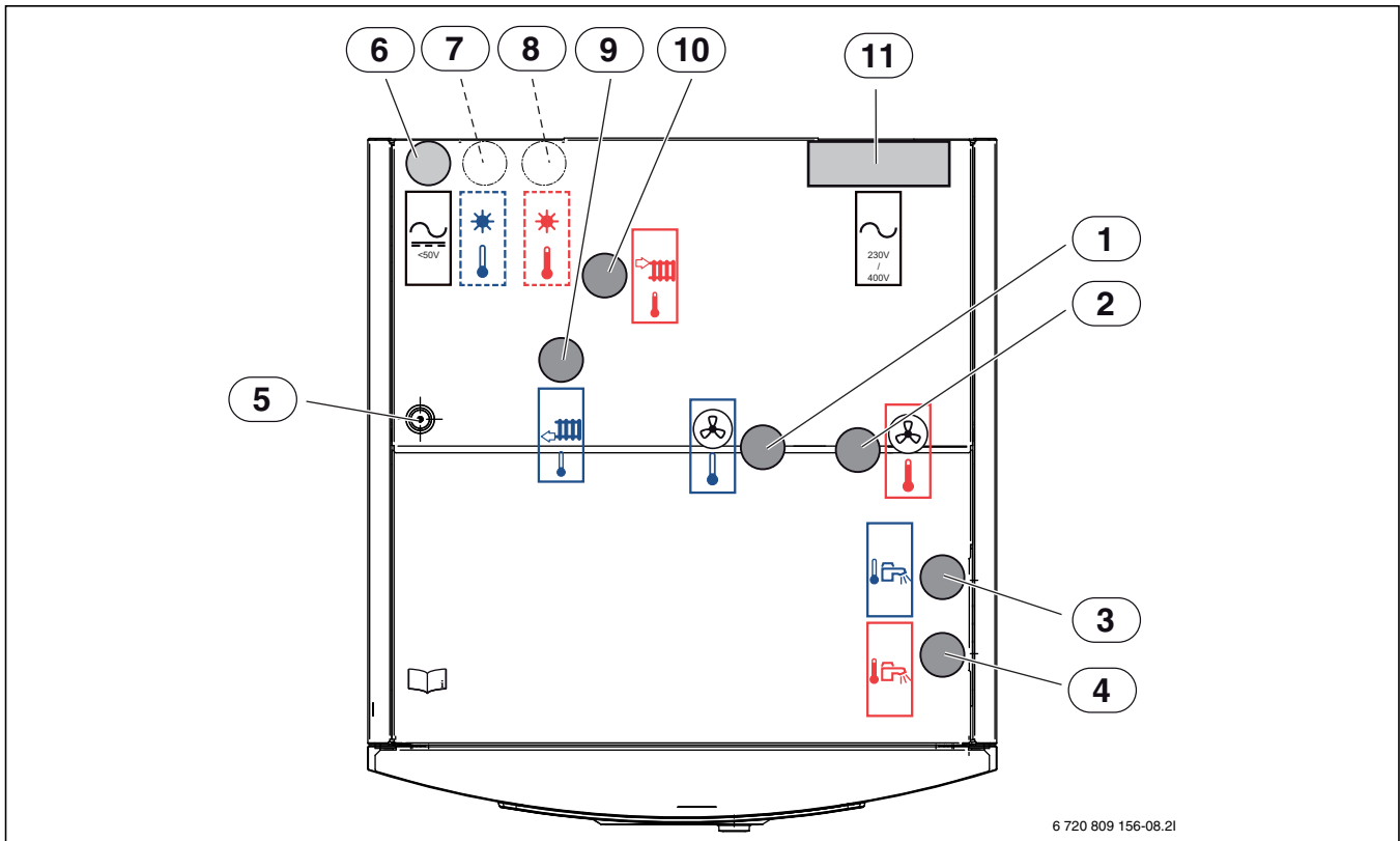
Kuva 8 Lämpöpumpputuulin liitännät
