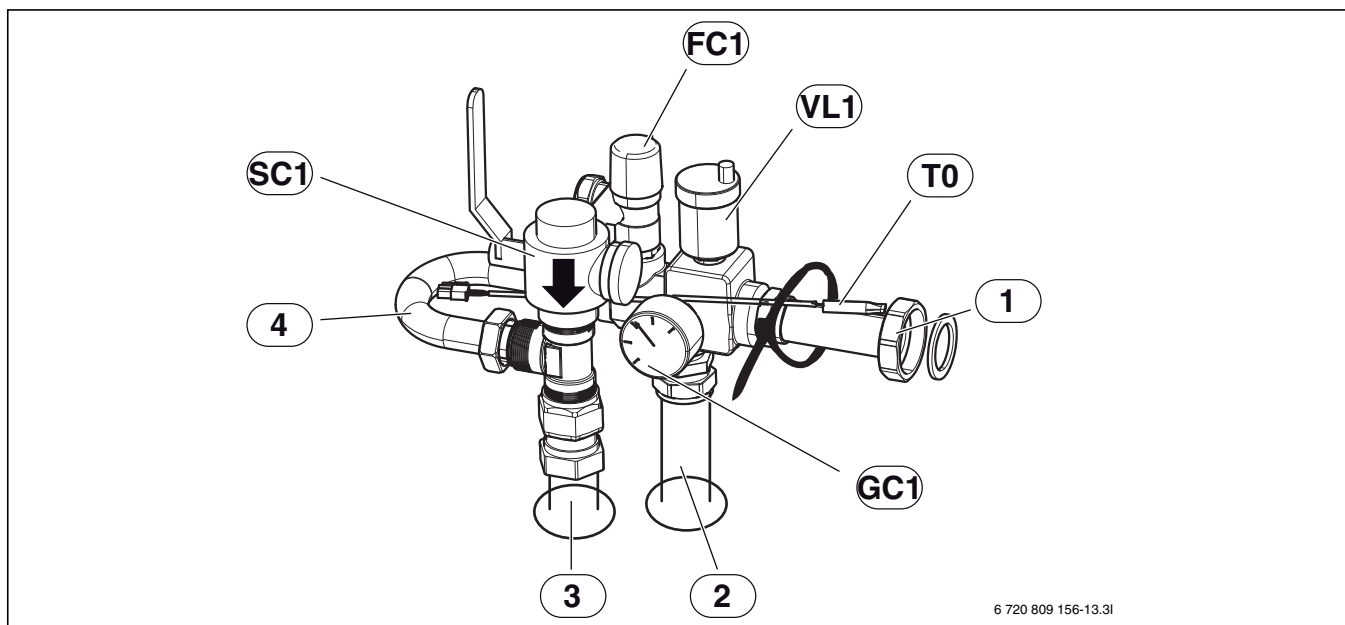
Kuva 10 Asennettu varoryhmä
