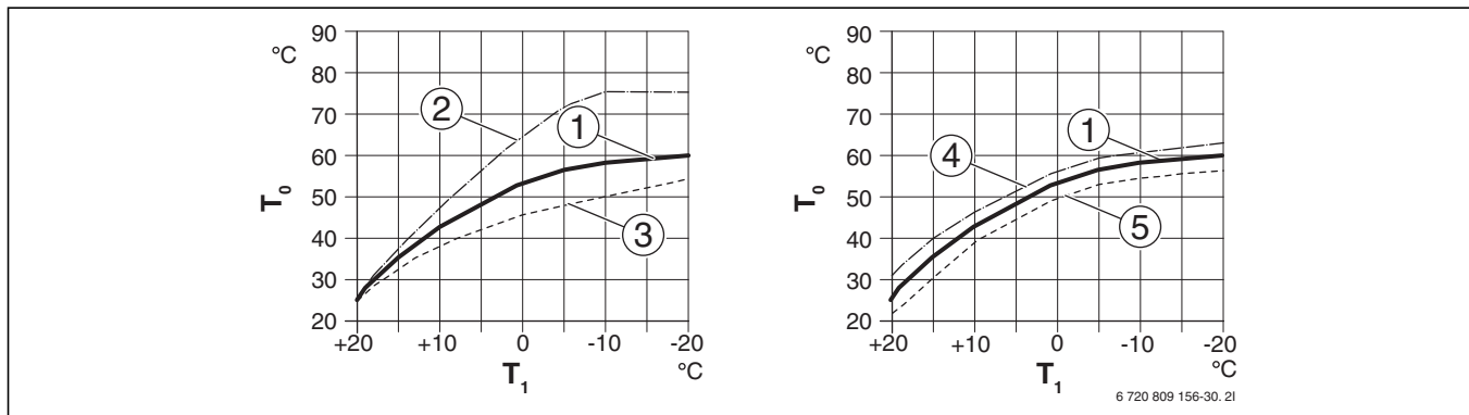
Kuva 40 Lämpöpatterien lämpökäyrä
