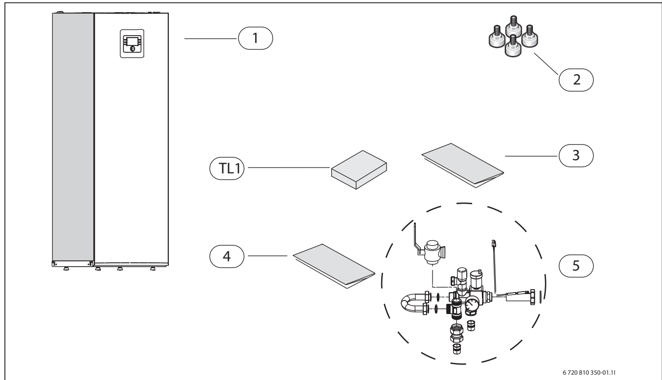
Kuva 1 Lämpöpumpputuuli
