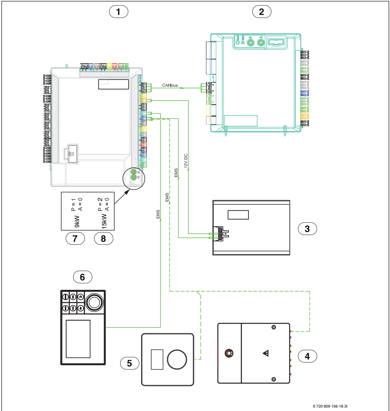
Kuva 31 Piirikaavio, lämpöpumppu/lämpöpumppumoduuli
