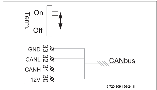
Kuva 17 CAN-väylän terminointi
