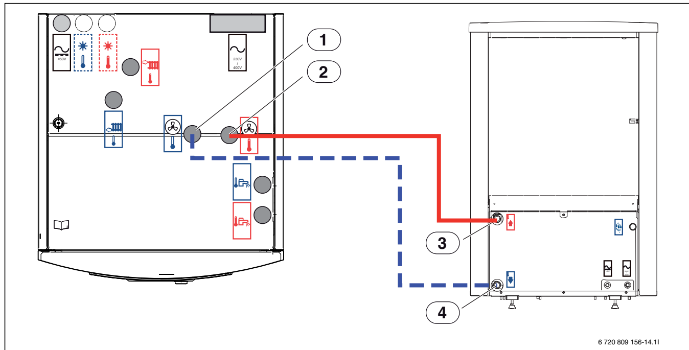
Kuva 11 Lämpöpumppumoduulin lämpöpumppuliitännät
