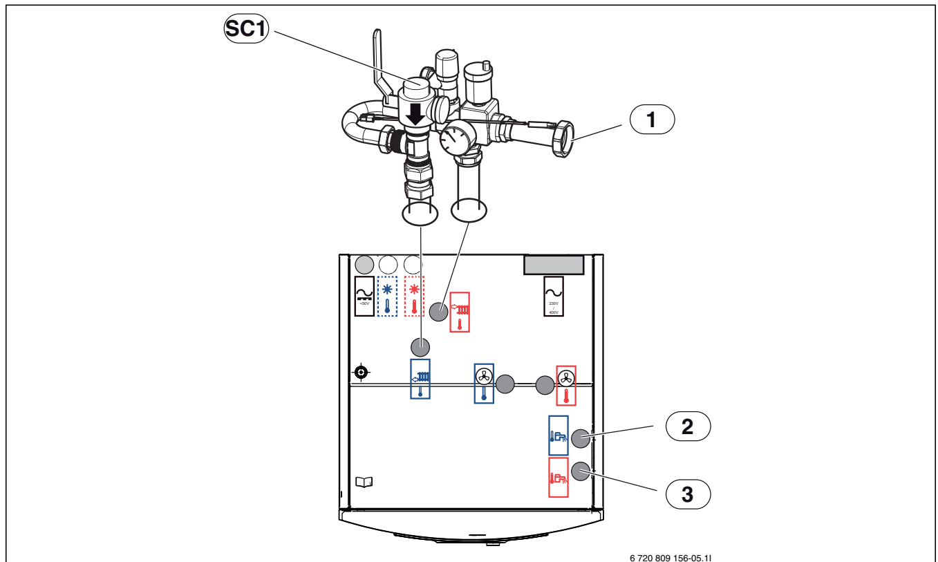
Kuva 12 Lämpöpumppumoduulin lämmitysjärjestelmä- ja käyttövesiliitännät
