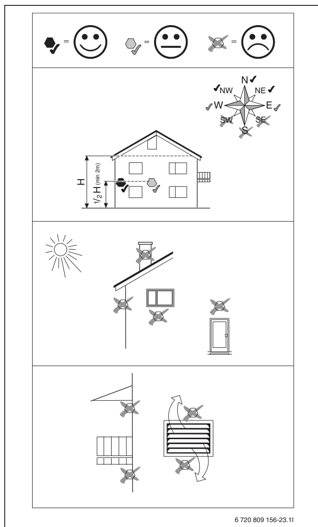
Kuva 15 Ulkolämpötila-anturien sijoittaminen
