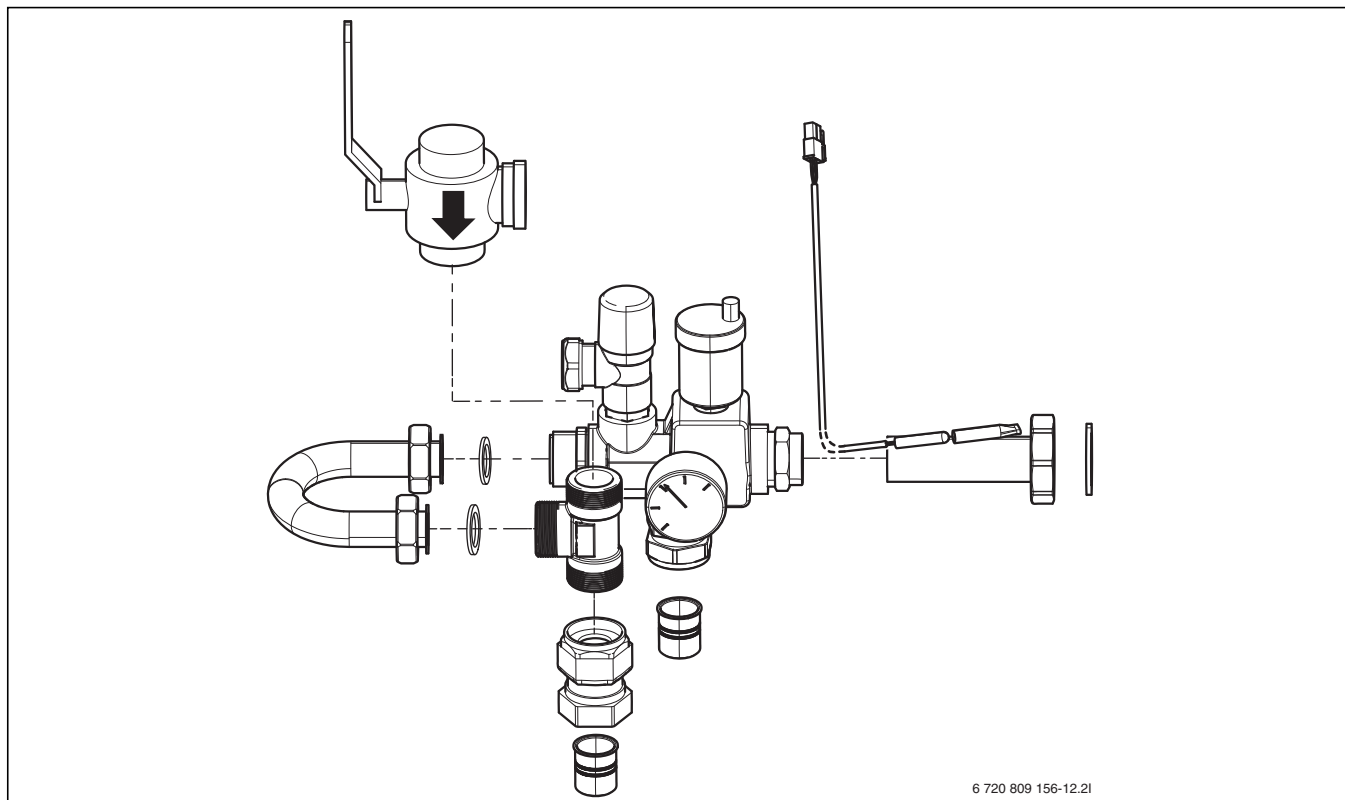
Kuva 9 Varoryhmän toimitusversio
