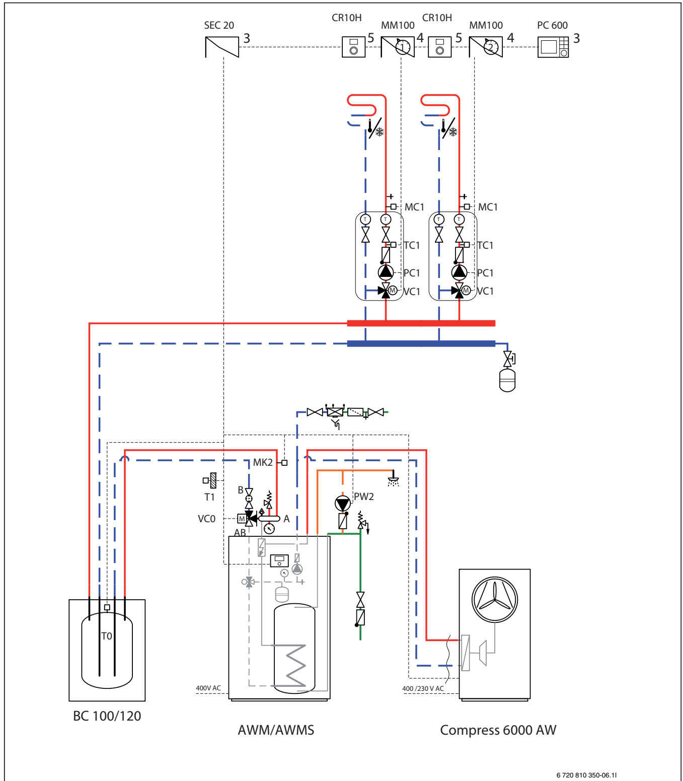
Kuva 4 Lämpöpumppu, lämpöpumppumoduuli ja puskurisäiliö
