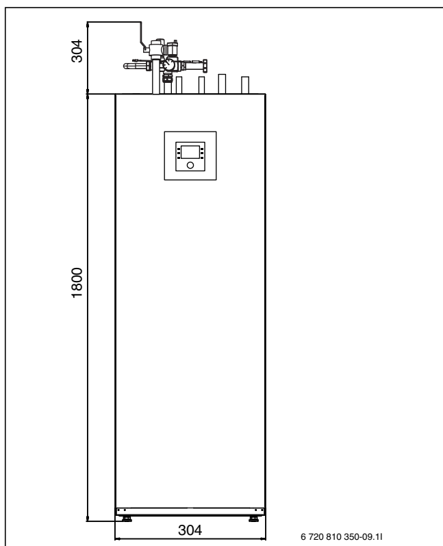
Kuva 6 Lämpöpumpputuotteen mitat (mm)
