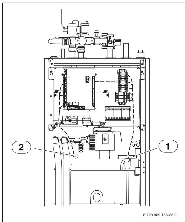
Kuva 19 Johtojen läpivienti
