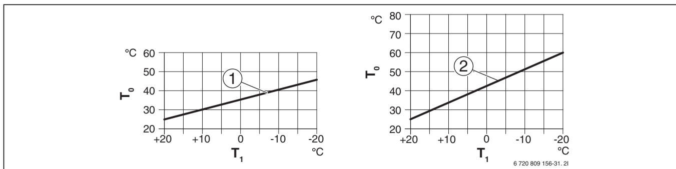
Kuva 41 yksinkertainen lämpökäyrä
