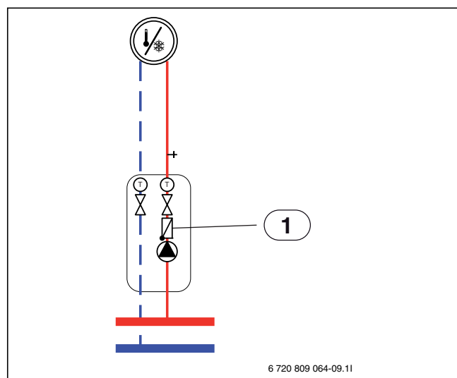
Kuva 2 Lämmityspiiri
