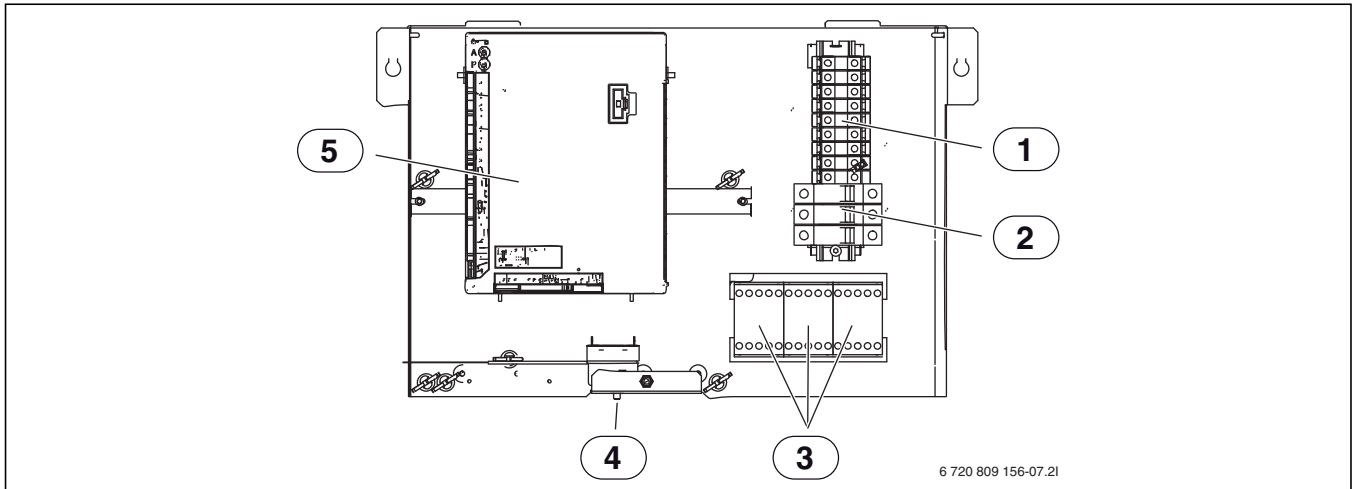
Kuva 20 Sähkökaapin malli
