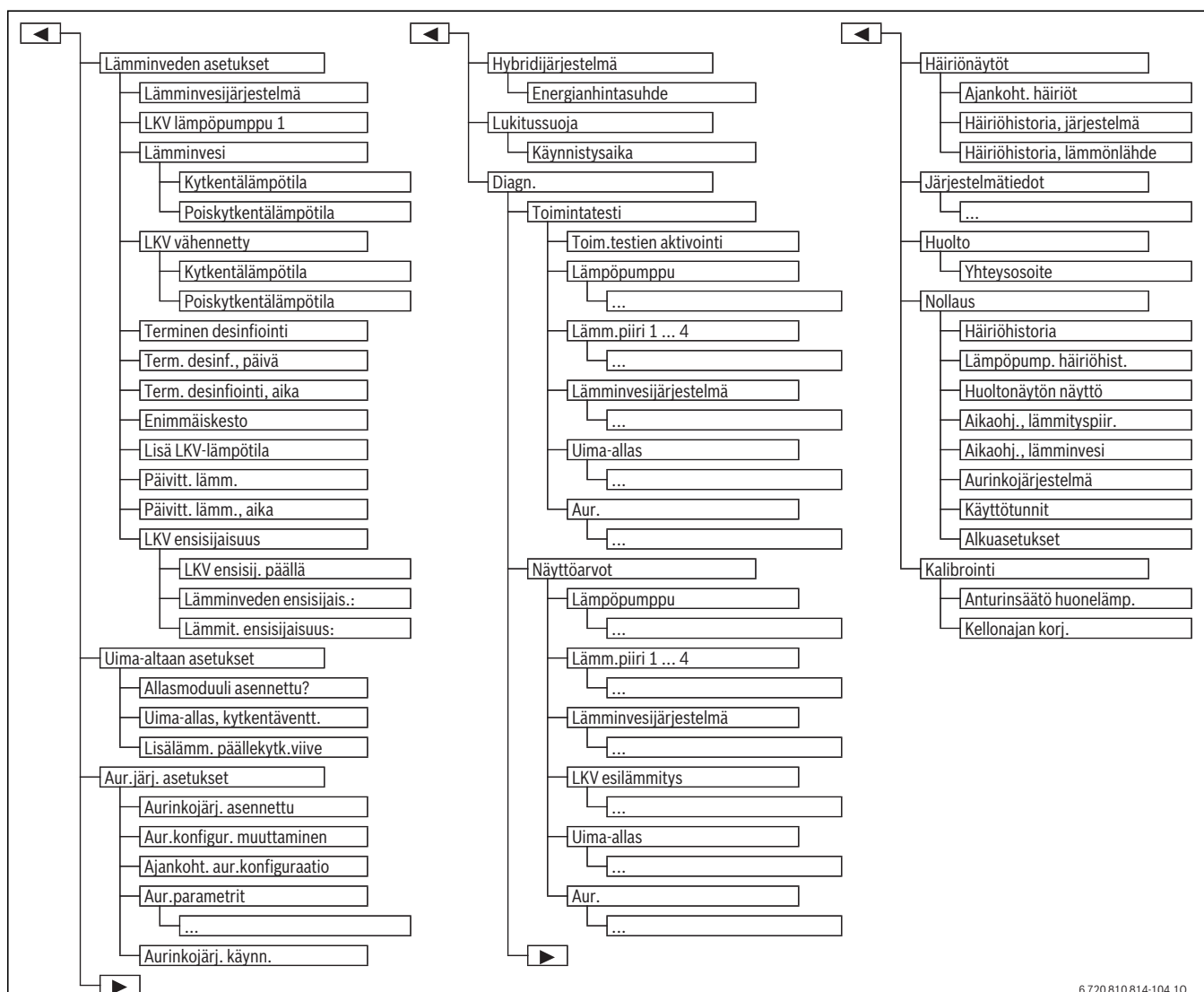
Kuva 36 Huoltovalikko 2/2
