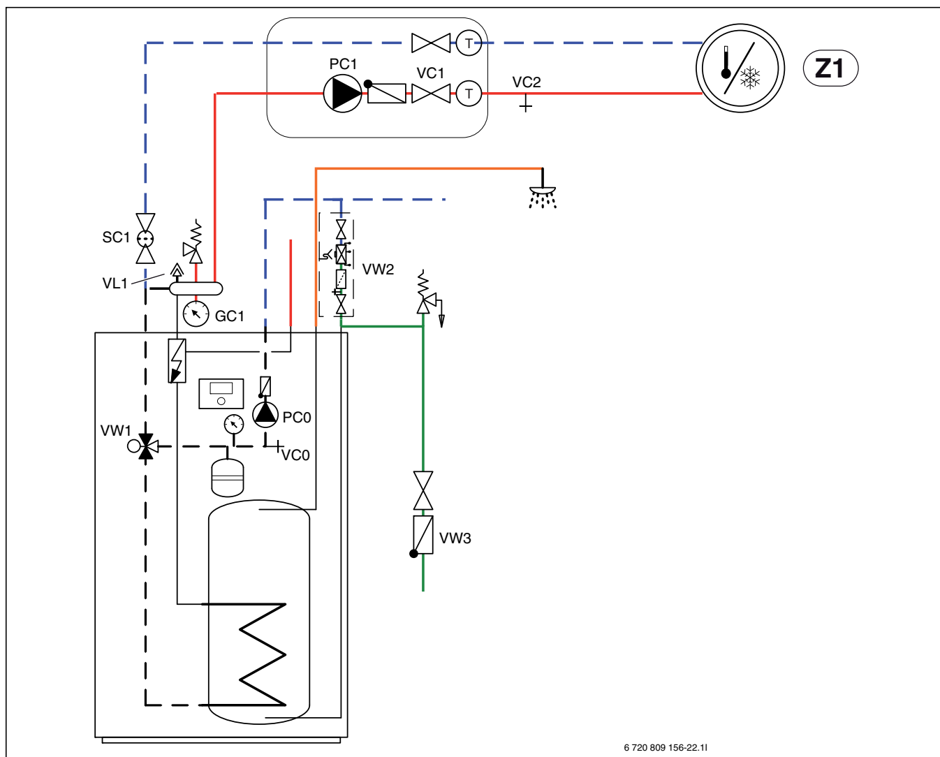
Kuva 16 Lämpöpumpputuotteen ja lämmitysjärjestelmä
