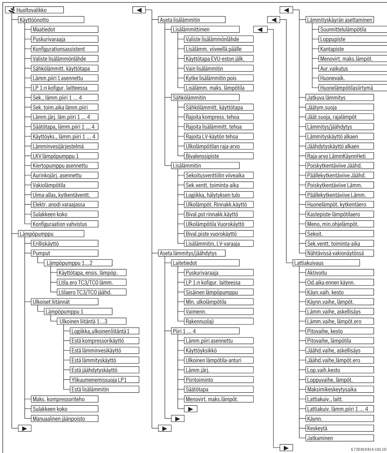
Kuva 35 Huoltovalikko 1/2
