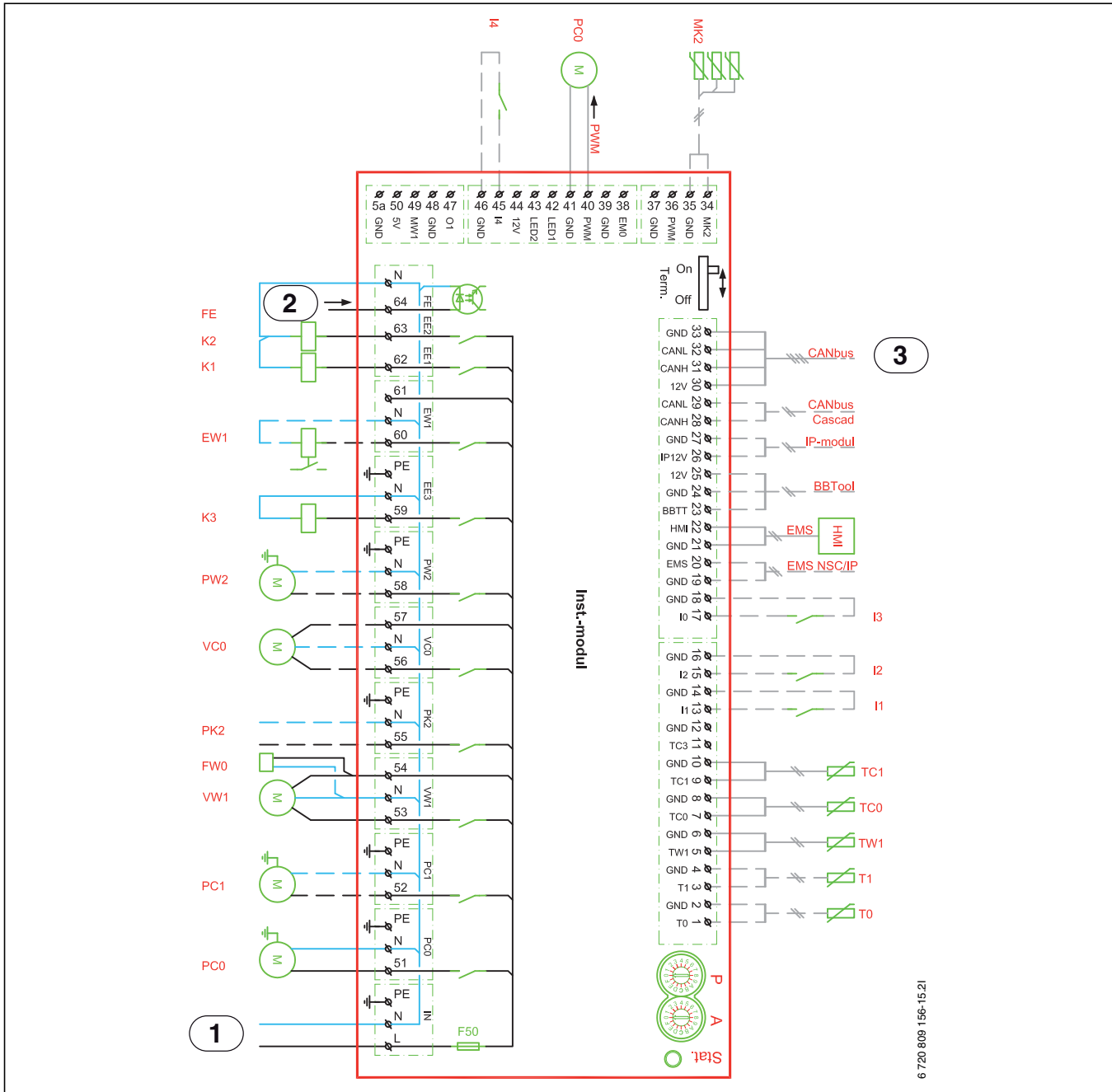
Kuva 30 Kytkentäkaavio, asennusmoduuli
