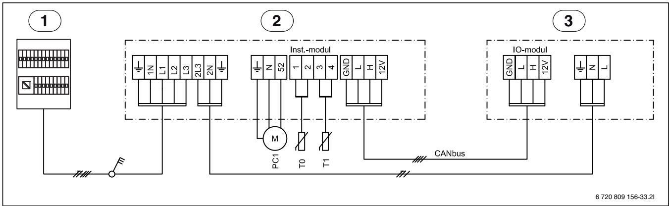
Kuva 24 Kytentäkaavio 9 kW 3N~
