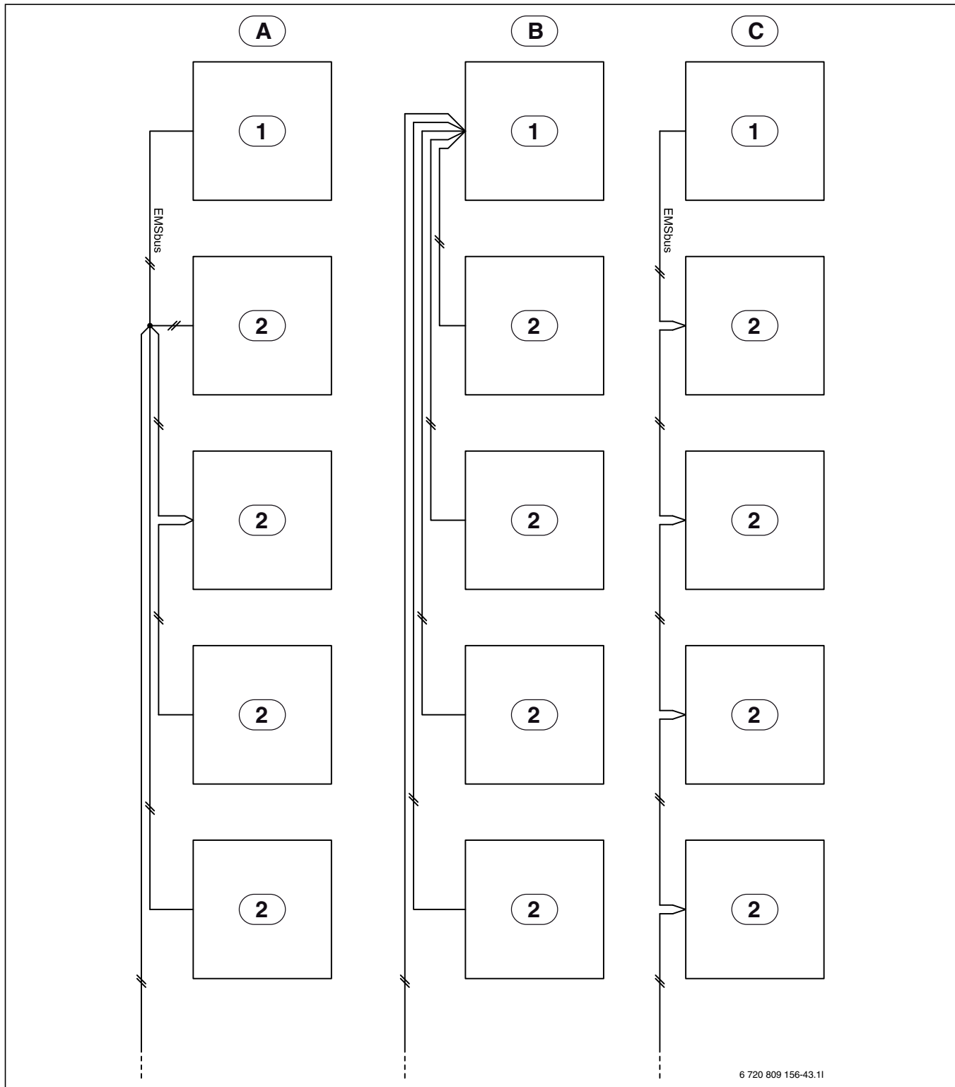
Kuva 32 Kytchentävaihtoehto, EMS-väylä
