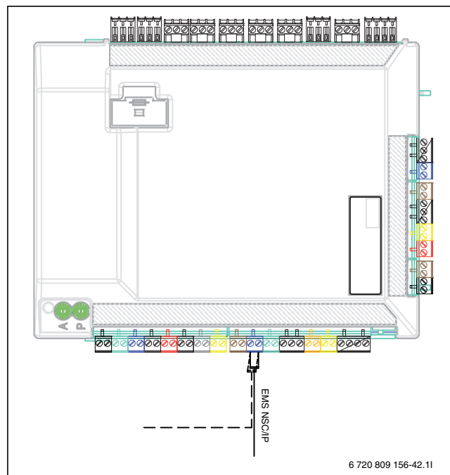
Kuva 14 Asennusmoduulin EMS-liitännät
